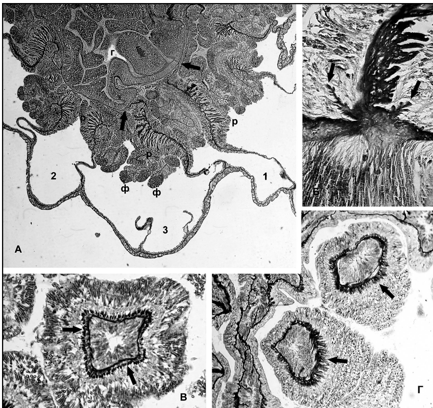
Рис. 3 Diadumene lineata : А – поперечный срез через колумену на уровне глотки, цифрами показаны пары мезентериев 3 порядков, мезентерии 1-го порядка прирастают к стенке глотки (показано стрелками), г – глотка, р – ретракторы, ф – филламенты; Б – срез через педальный диск, стрелками указаны базилярные мускулы; В – поперечный срез через верхнюю часть щупальца, стрелками показана продольная эктодермальная мускулатура; Г – поперечный срез через верхнюю часть колумены, видны поперечные срезы через основания щупалец, где эктодермальная мускулатура сильнее (стрелки)
